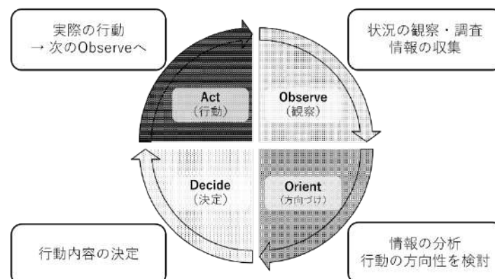
図 14 OODA ループ
